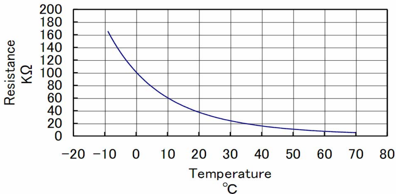
热敏电阻的温度曲线图
